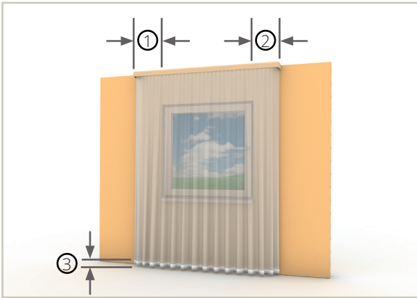
Abb.1 1. Überlappung der Gardinenstange / -schiene links 15-30 cm 2. Überlappung der Gardinenstange / -schiene rechts 15-30 cm 3. Bodenabstand Gardine ca. 1,0 cm
